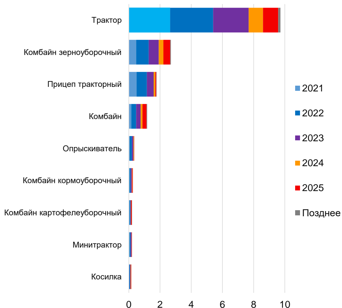
Сельскохозяйственная техника, тыс. ед., по годам завершения действия договоров*
